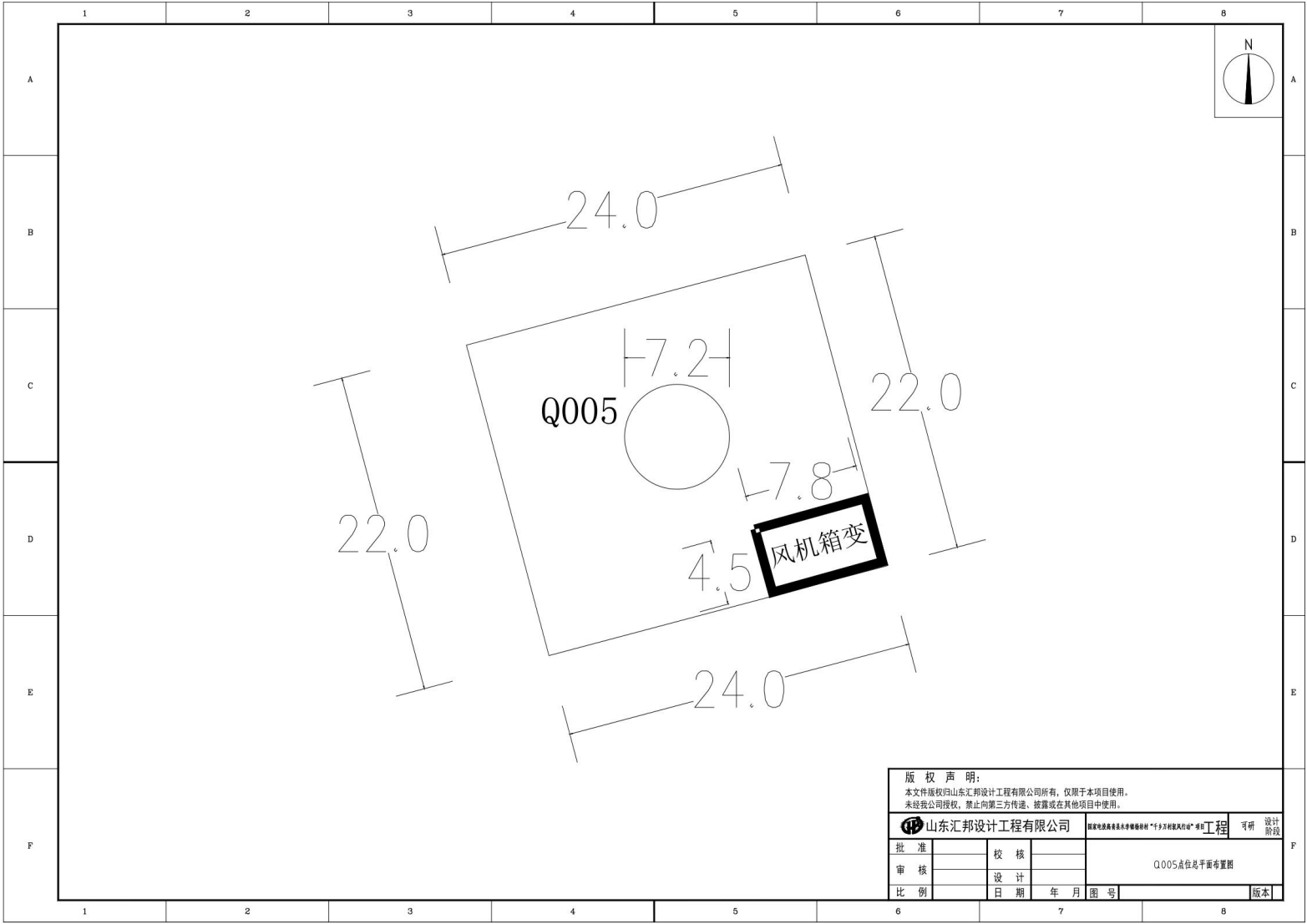
附图 3b：项目风机平面布置图
