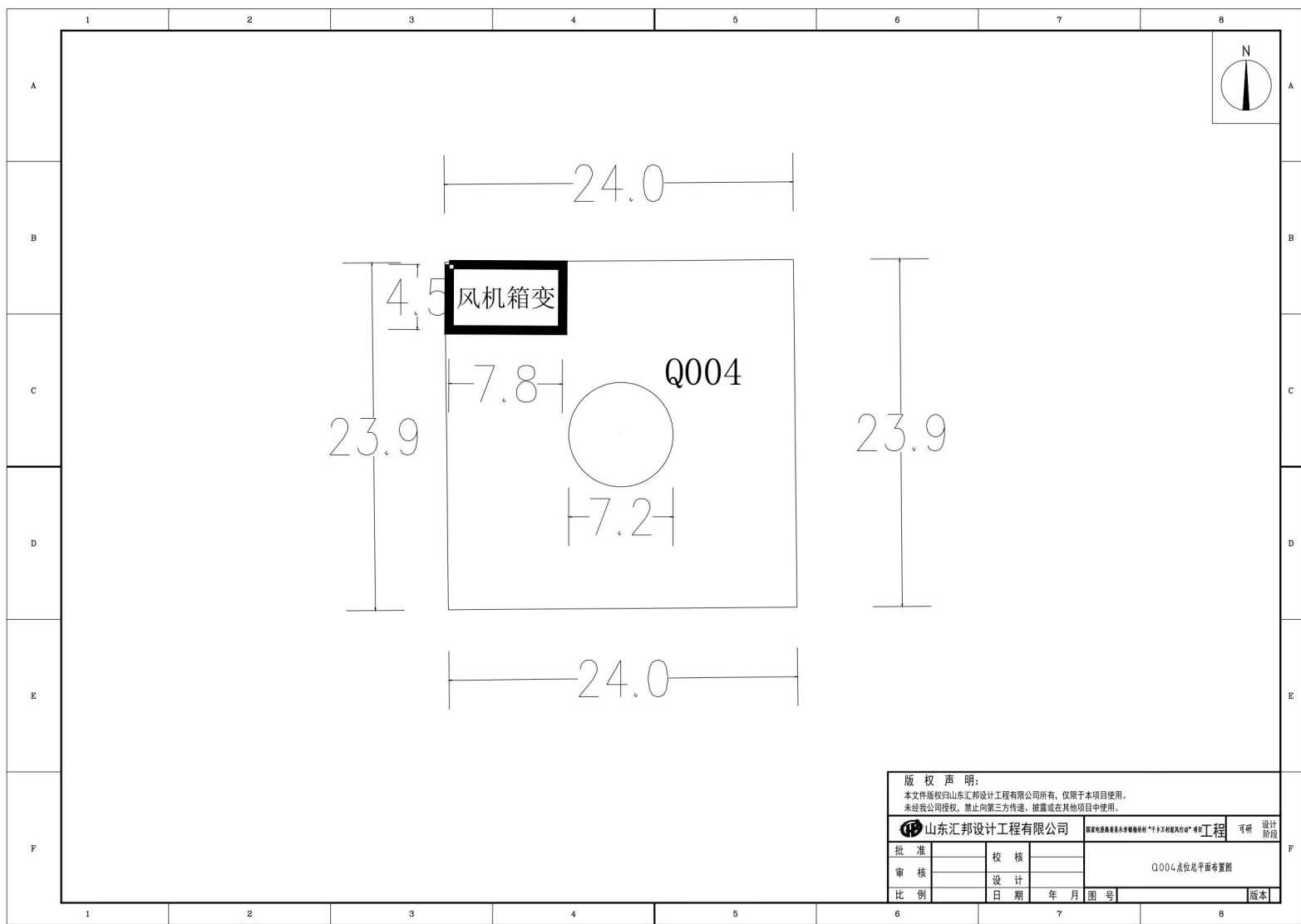
附图 3a: 项目风机平面布置图
