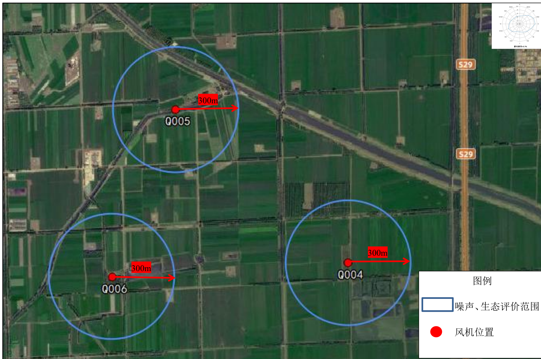
附图 8a: 项目评价范围图
