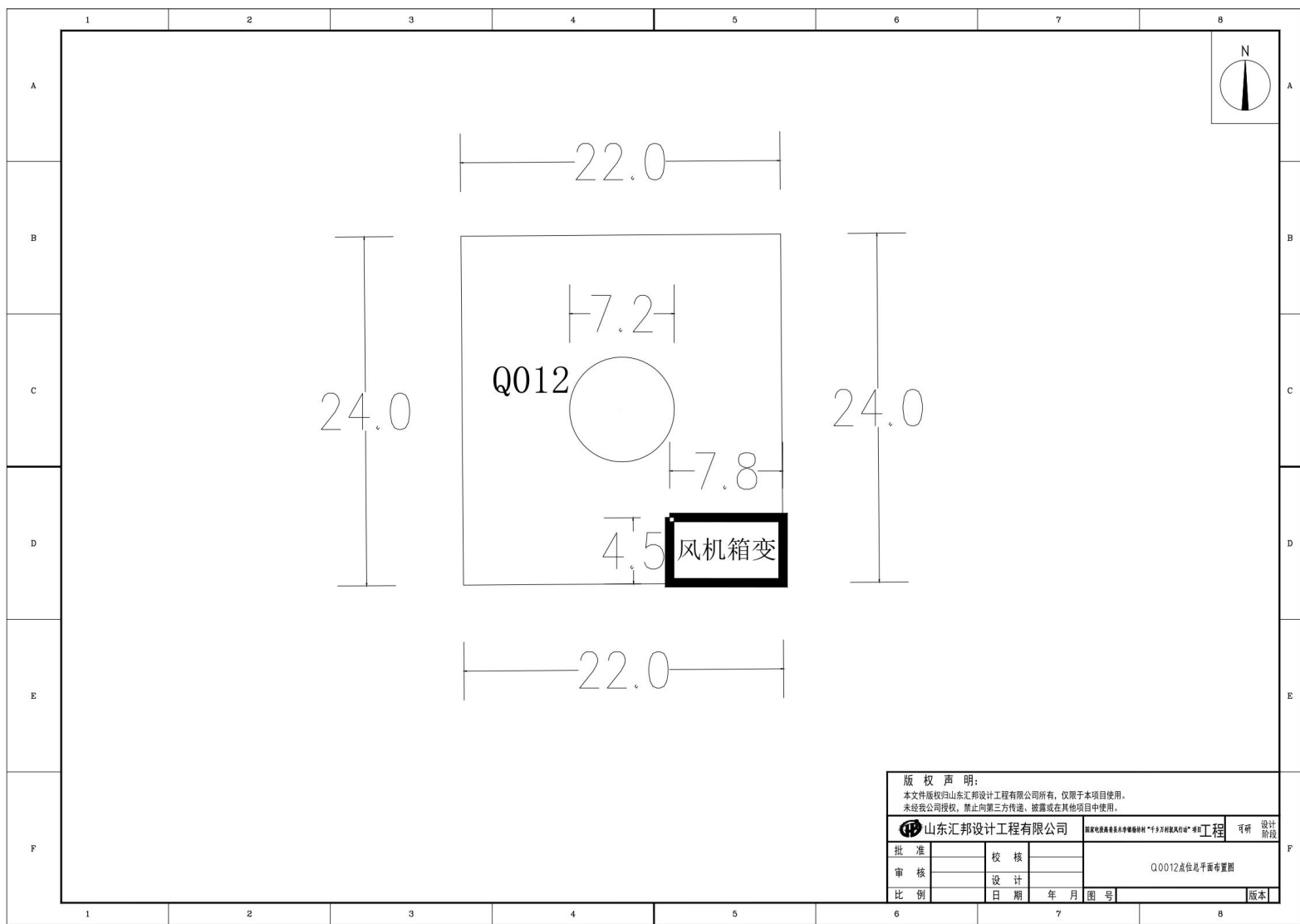
附图 3i：项目风机平面布置图
