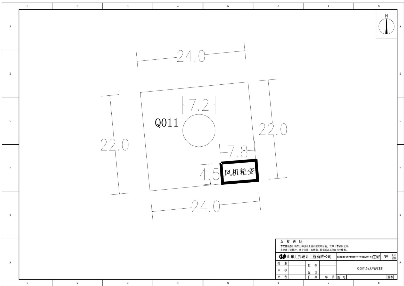
附图 3h：项目风机平面布置图
