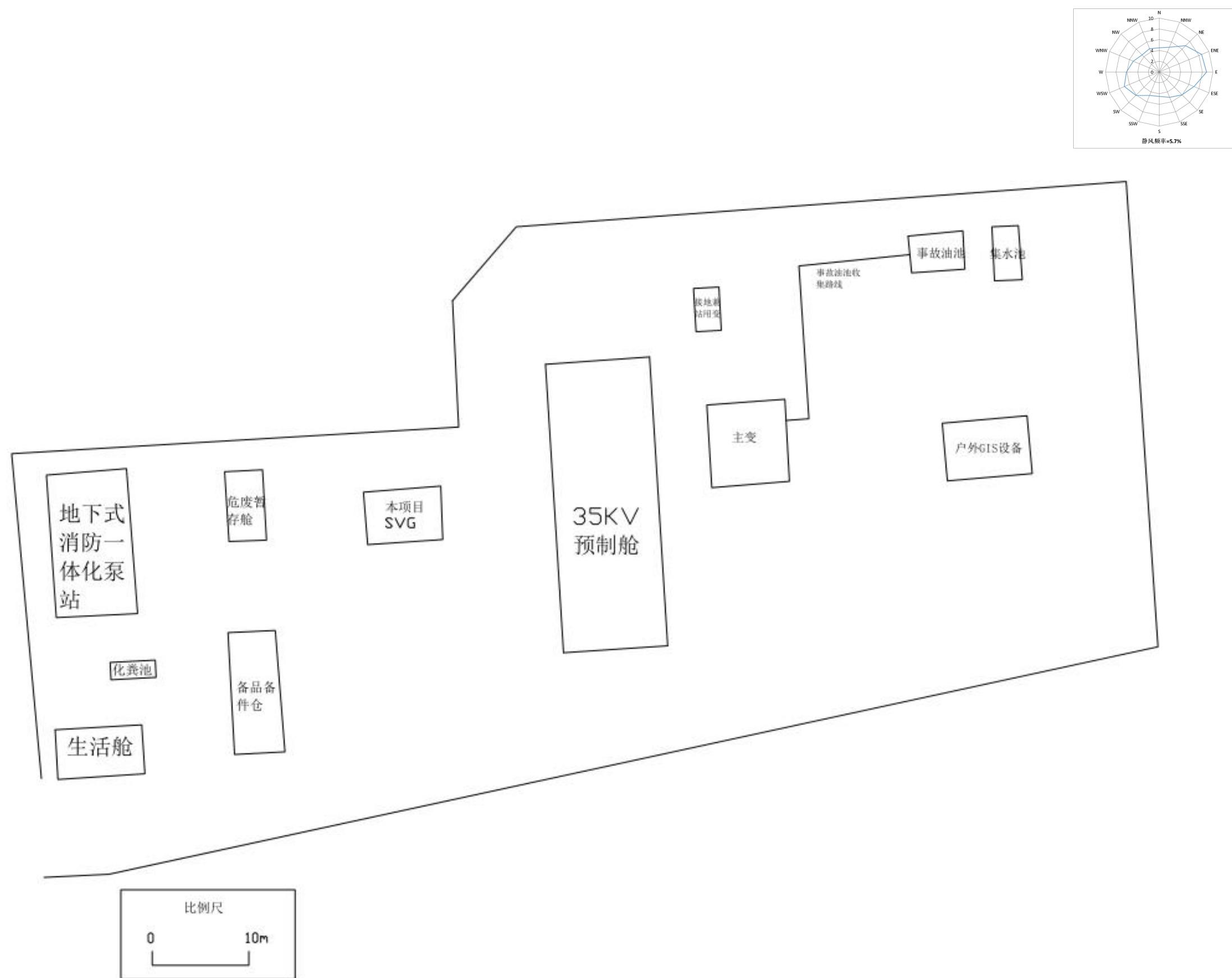
附图 3j: 升压站平面布置图
