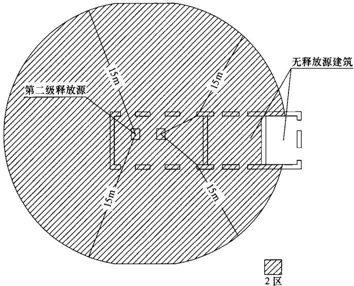
图 E.0.5 与具有第二级释放源的建筑物相邻，并采用不燃烧体实体墙隔开时，其爆炸危险区域和范围划分的
